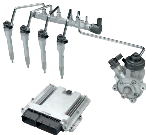
Abb. 11: Exemplarische Darstellung eines Einspritzsystems am Beispiel eines Diesel Common-Rail-Systems (Quelle: Bosch)
