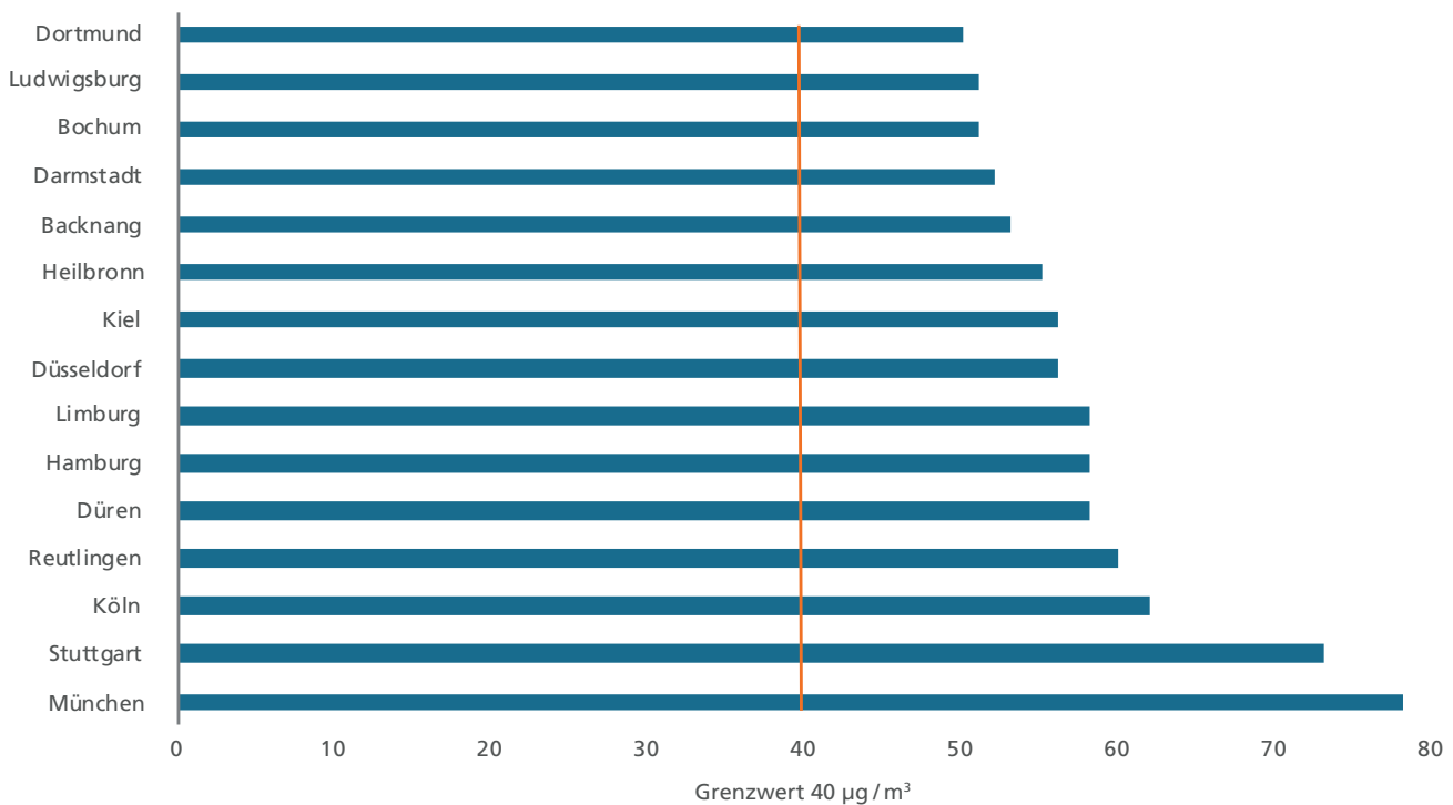
Abb. 3: Die 15 Städte mit den höchsten NO 2 -Grenzüberschreitungen 2017 (UBA, 2018)
